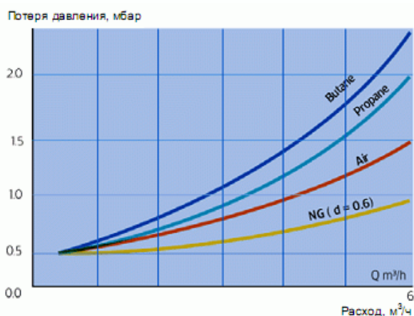
Потери давления счётчика Gallus 2000 (Галлус 2000)
